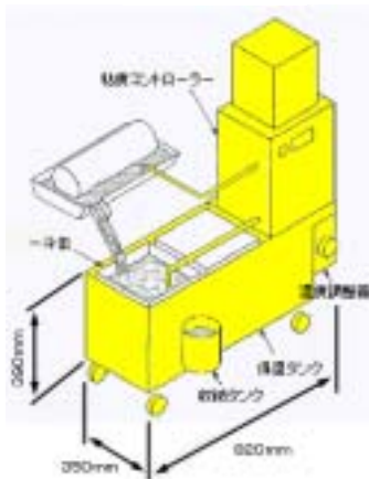
〔設置例図〕
